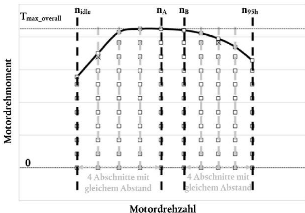
Abbildung 1 Bestimmung der Drehzahleinstellpunkte
