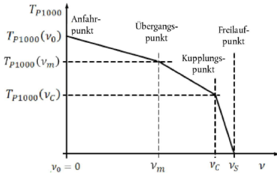
Abbildung 2 Allgemeines Drehmomentverhältnis
