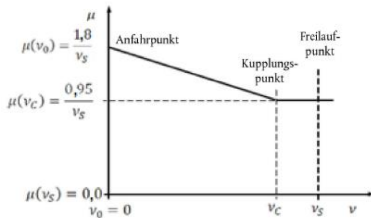
Abbildung 2 Allgemeines Drehmomentverhältnis
