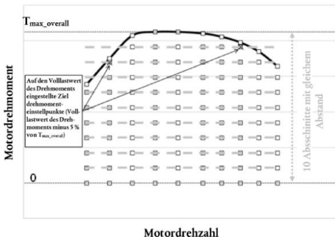
Abbildung 2 Bestimmung der Drehmomenteinstellpunkte
