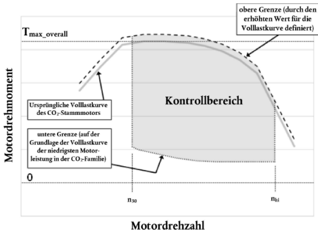
Abbildung 5 Beispielhafte Bestimmung der Motordrehzahl-, Motordrehmoment- und Motorleistungsbereiche für den Kontrollbereich
