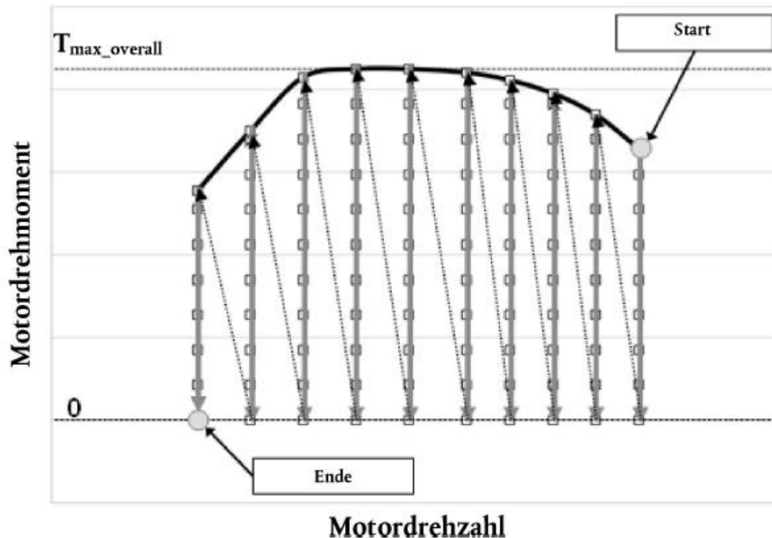
Abbildung 4 Sequenz der stabilen Messeinstellpunkte
