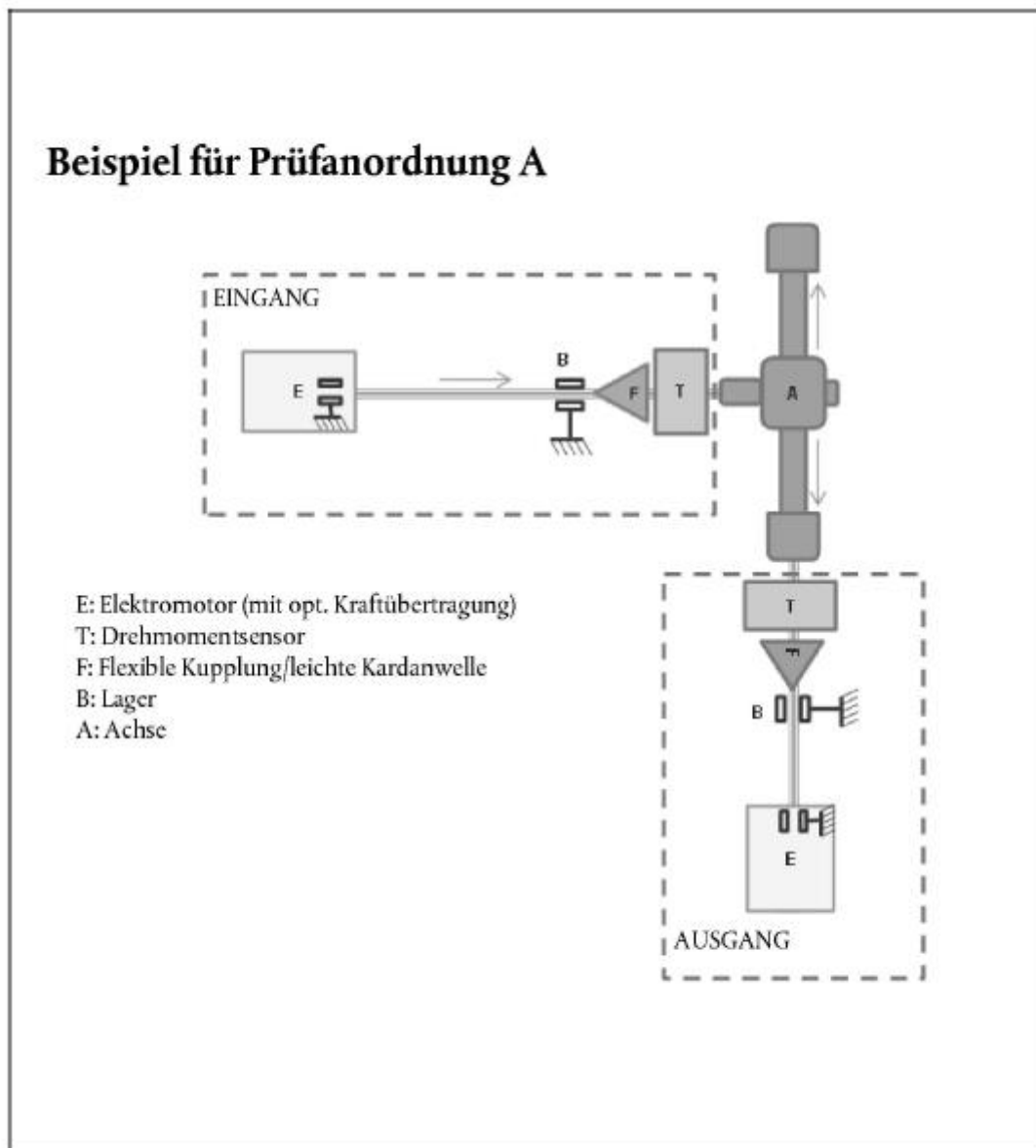
Abbildung 1 Beispiel für eine Prüfanordnung „Typ A“
