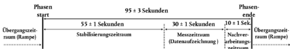
Abbildung 3 An den einzelnen Messeinstellpunkten auszuführende Schritte
