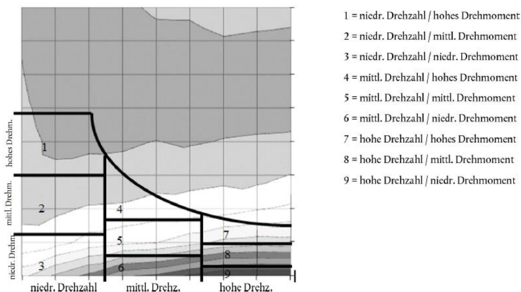
Abbildung 2 Drehzahl- und Drehmomentbereiche zur Überprüfung der Übereinstimmung der für die CO 2 -Emissionen und den Kraftstoffverbrauch maßgeblichen zertifizierten Eigenschaften
