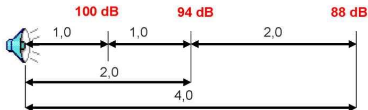
Abb. 3 Schallpegelabnahme im Freien um 6 dB je Abstandsverdopplung
