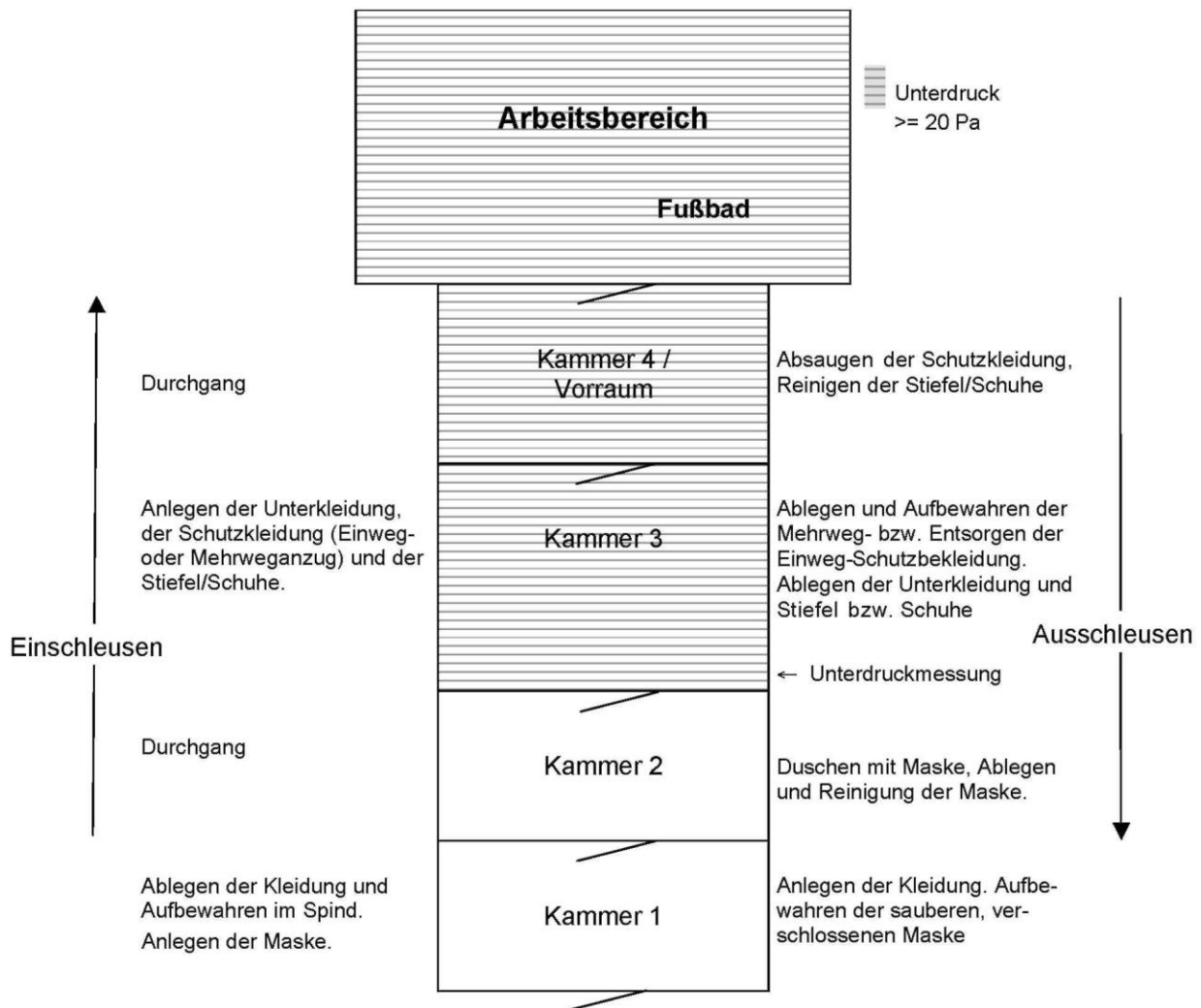
Abb. 1 Personenschleuse(Prinzipskizze)
