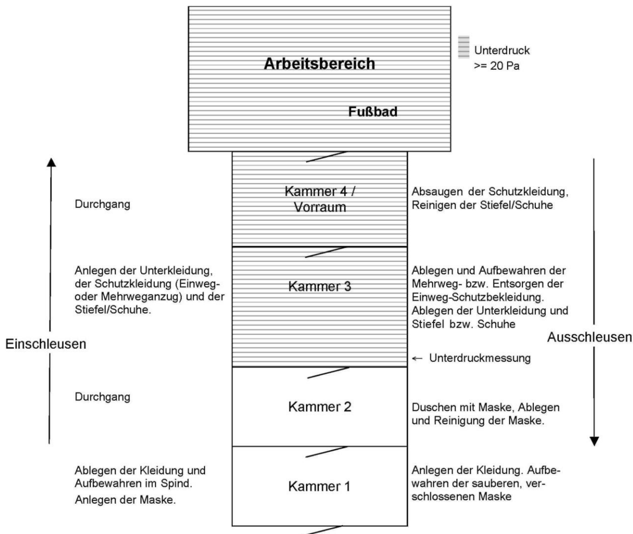
Abb. 1 Personenschleuse(Prinzipskizze)
