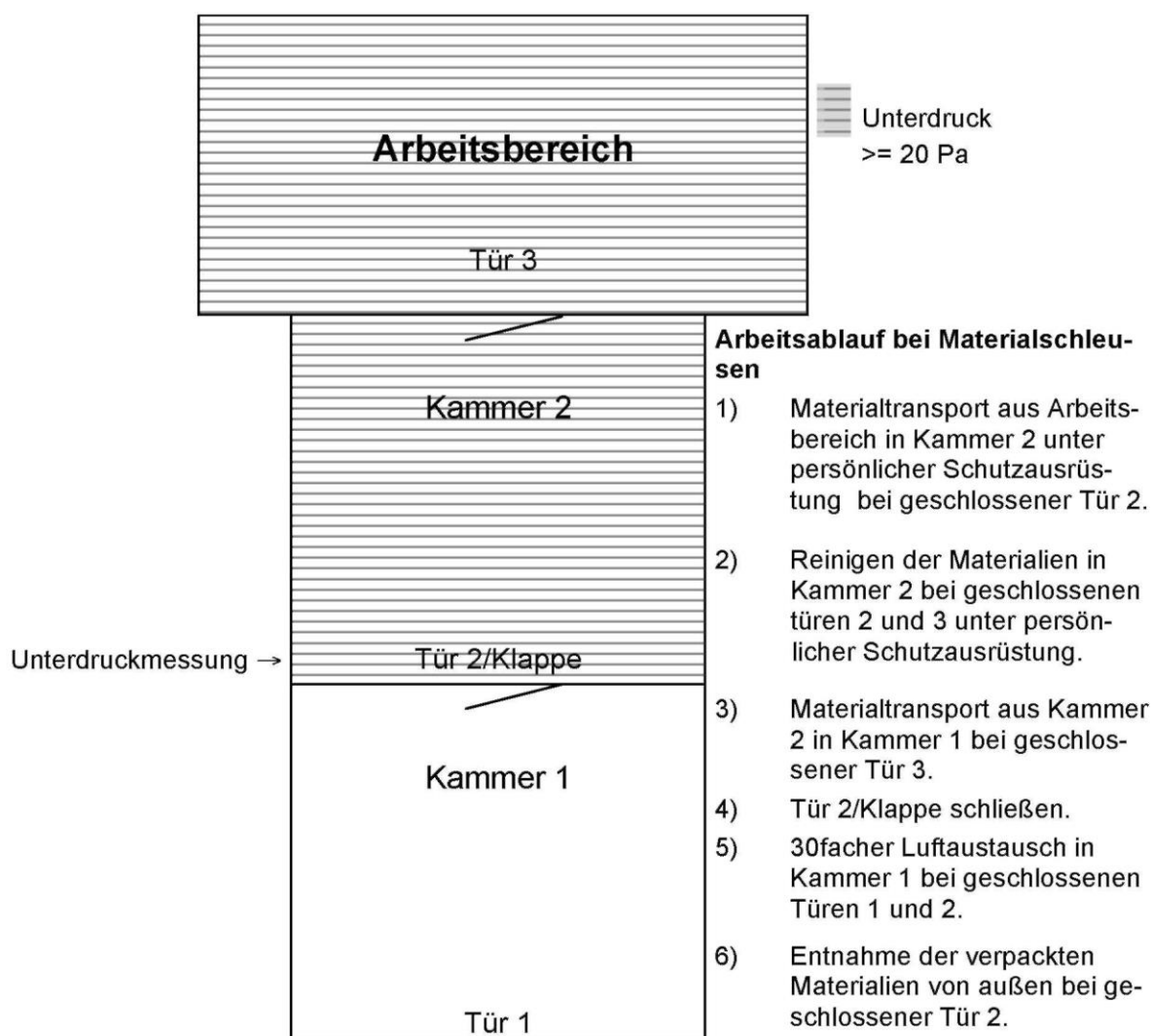
Abb. 2 Materialschleuse (Prinzipskizze)
